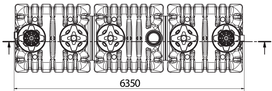
Epurbloc 185 12000 | 13230120
