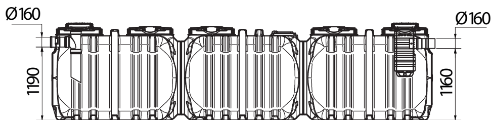
Epurbloc 185 12000 | 13230120
