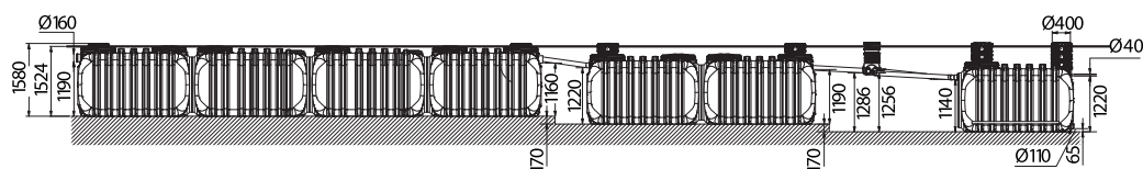
Actifiltre 185 30000-20000 | 1380E301
