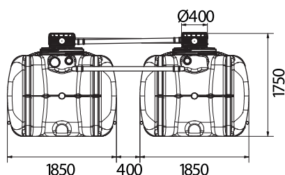
Actibloc 185 6000-6000 | 1370E014
