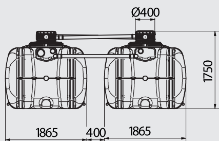
Actibloc 185 10000-10000 | 1370E030
